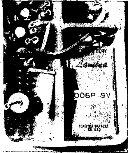
Un transmisor instalado en una jabonera de plástico. A su lado se ve una bobina de fabricación casera.
