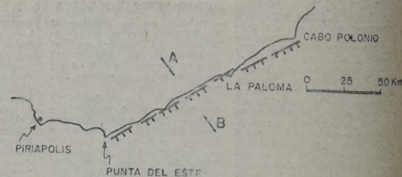
Estudios geológicos de la costa de Maldonado y Rocha, que identifican sitios de posible acumulación de hidrocarburos, muestran que también en esta parte de la costa del Río de la Plata y Océano Atlántico el Uruguay tiene expectativas de explotación de petróleo.
